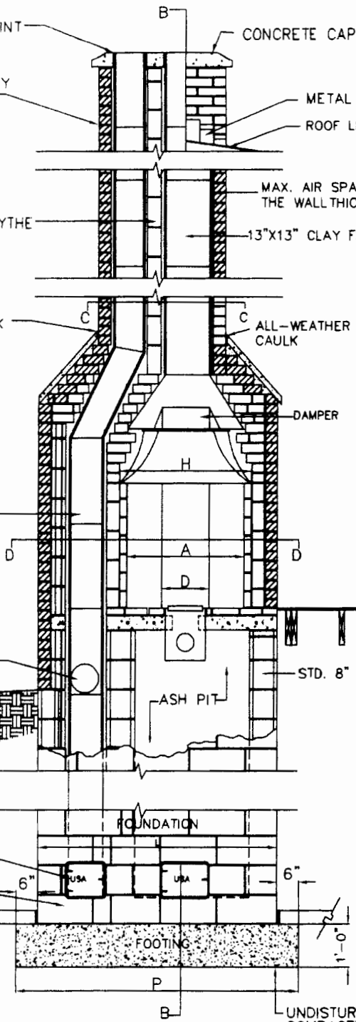
SECTION A-A
