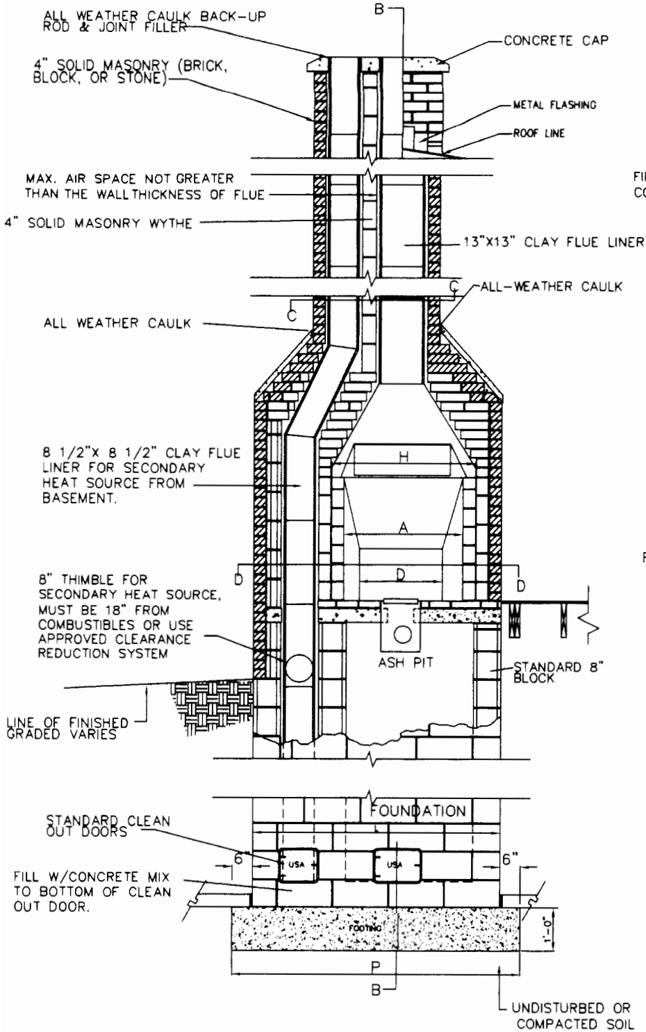
SECTION A-A
